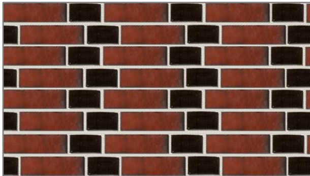
Gotischer Verband
