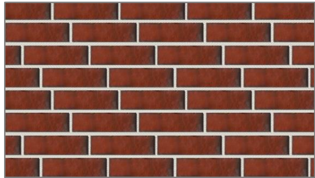
1/4-Steins-Läuferverband
