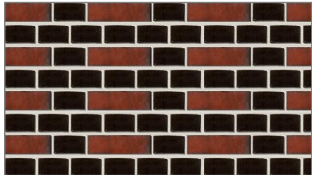
Holländischer Verband
