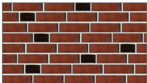
Wilder Verband
